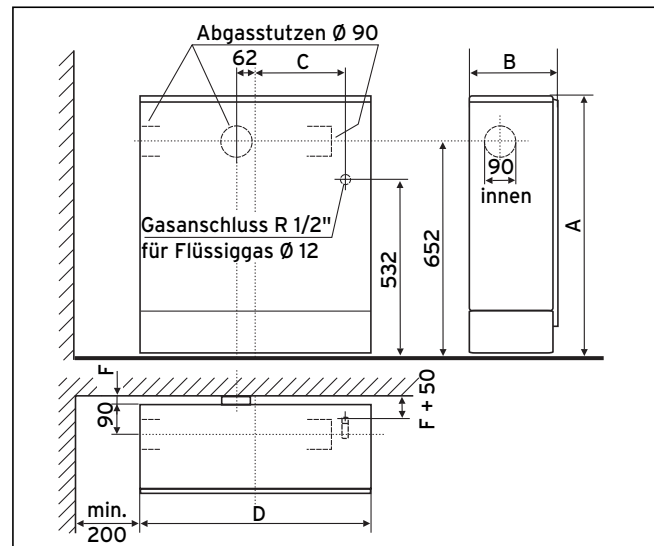
Abb. 5.1 Maßskizze VGR 30/4 X bis VGR 90/4 X
