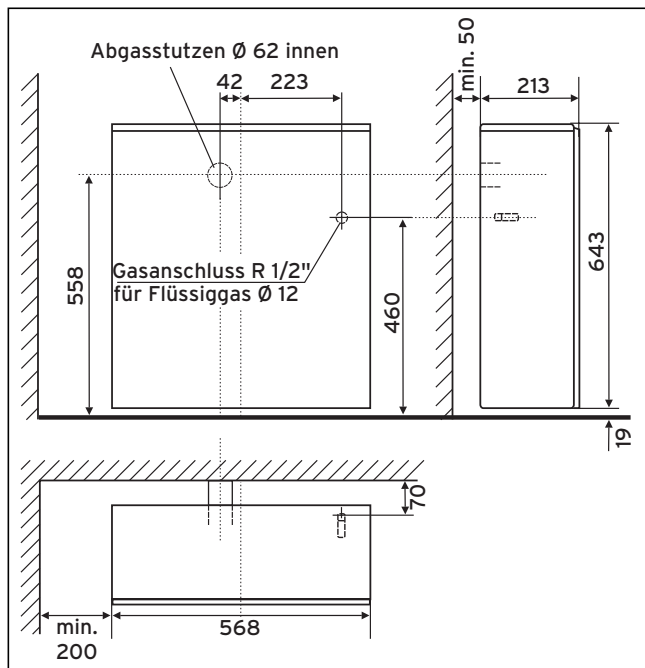
Abb. 5.2 Maße VGR 30 F/4 X
