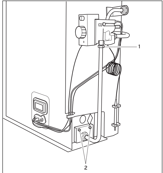
Abb. 7.1 Austausch der Hauptbrennerdüse
