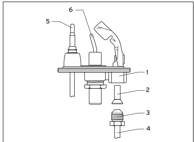
Abb. 7.3 Zündbrenner mit Anschlüssen
