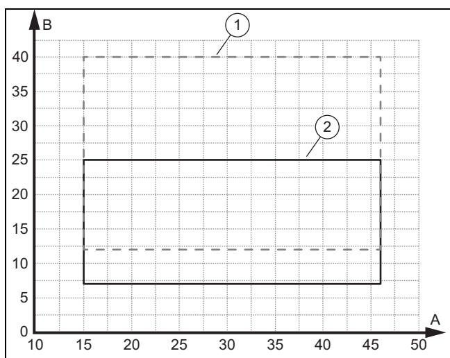
A Außentemperatur B Heizwassertemperatur 1 Einsatzgrenzen, Anlaufphase Kühlen 2 Einsatzgrenzen, Normalbetrieb Kühlen
