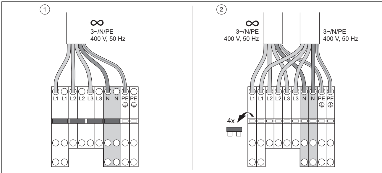
1 Einkreisschaltung mit permanenter Stromversorgung (3~/N/PE, 400 V, 50 Hz)
