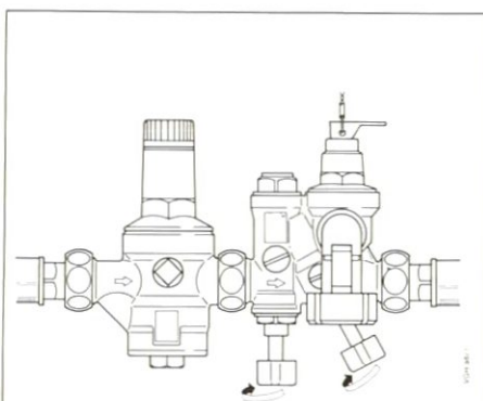
Abb. 1 Kaltwasser-Absperrventile öffnen
