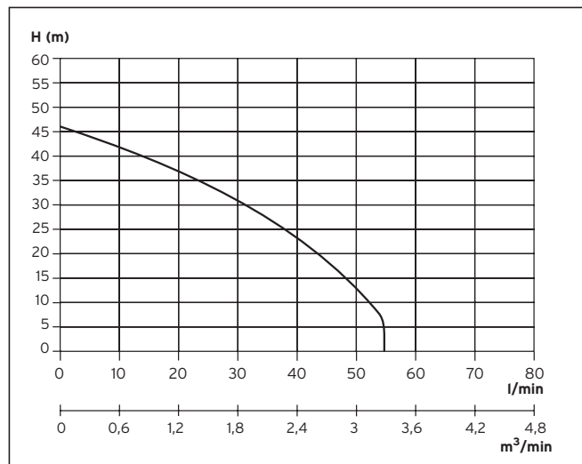
Abb. 4.1 Pumpenkennlinie
