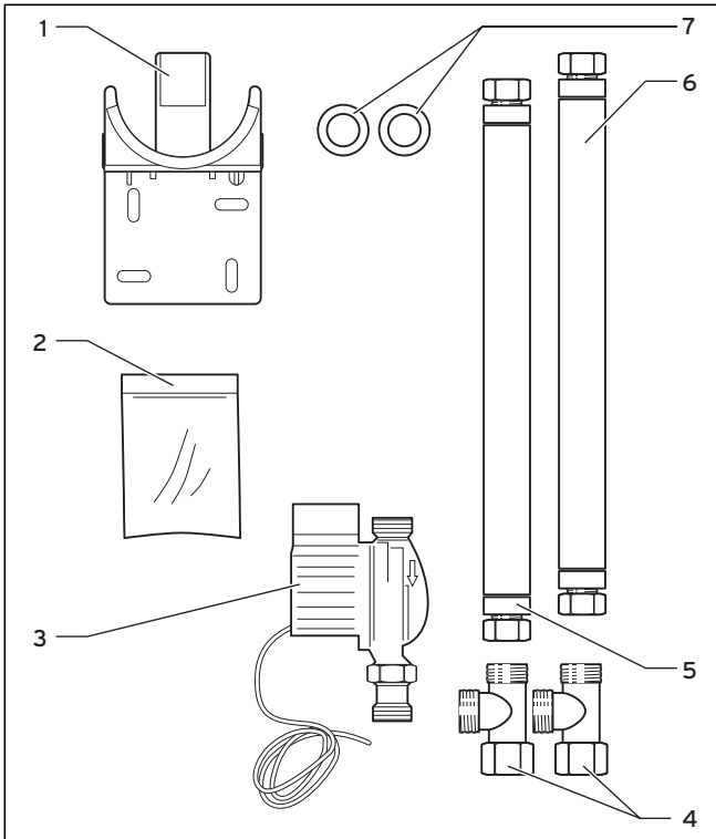
Abb. 2.1 Lieferumfang Legionellenschutzbaugruppe Art.Nr. 302 694
