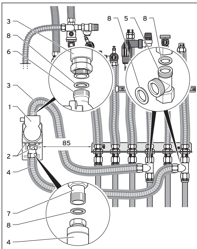
Abb. 3.2 Montage bei Anschlusskonsole Aufputz
