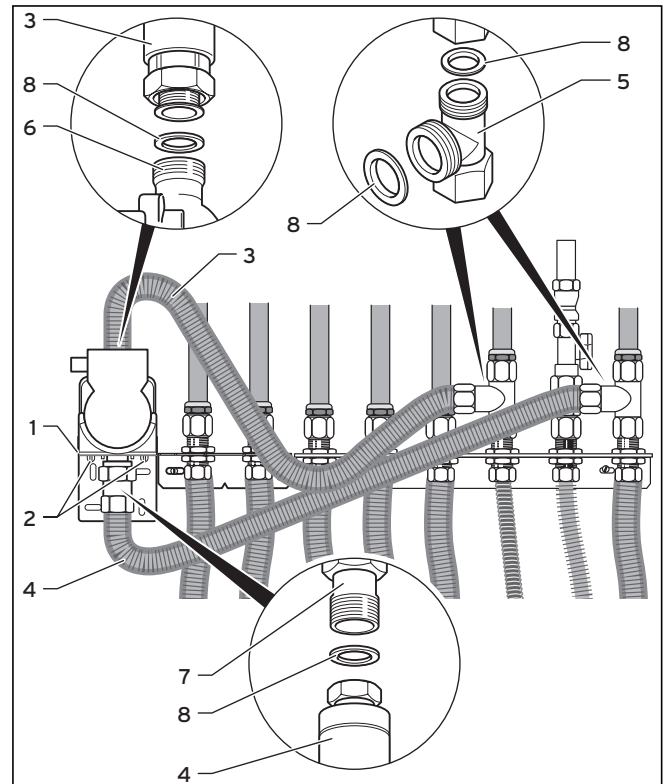
Abb. 3.1 Montage bei Anschlusskonsole für Installation von oben mit Solar-Anschlusskonsole
