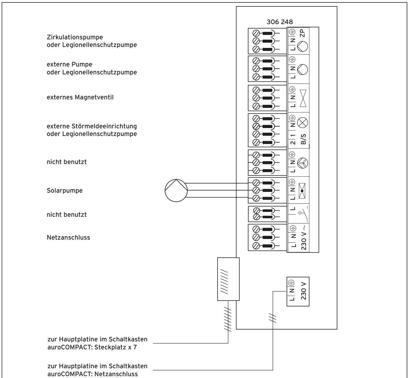
Abb. 3.3 Anschlussverdrahtung Zusatz-Anschlußbox (Zubehör, Art.-Nr.: 306 248)
