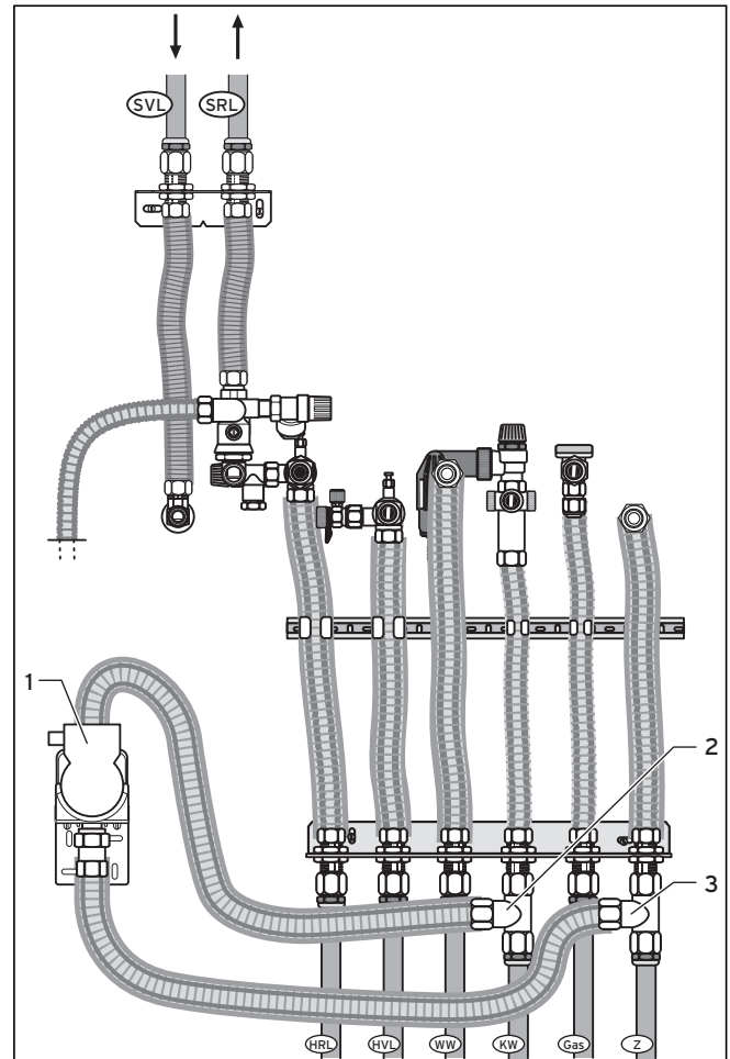
Abb. 1.2 Legionellenschutzbaugruppe in Verbindung mit Anschlusskonsole Aufputz
