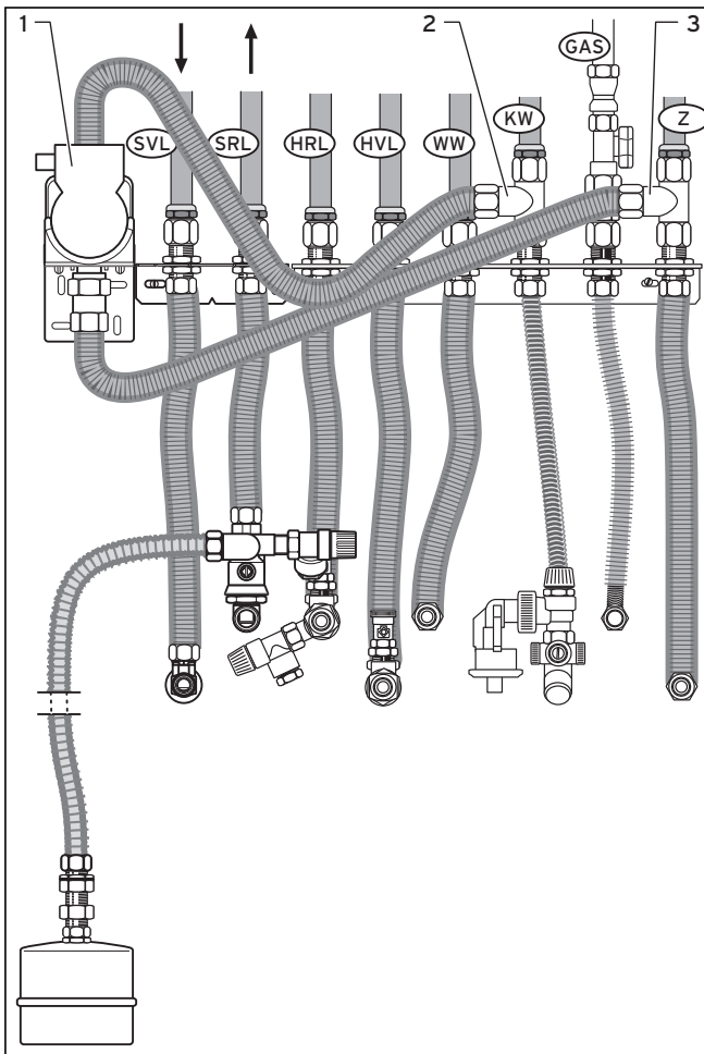
Abb. 1.1 Legionellenschutzbaugruppe in Verbindung mit der Anschlusskonsole für Installation von oben
